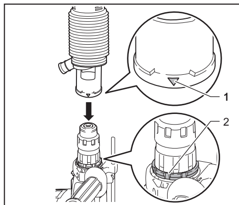
► 1. Capuchon à poussières
