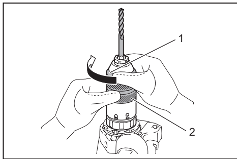
► 1. Sleeve 2. Ring
